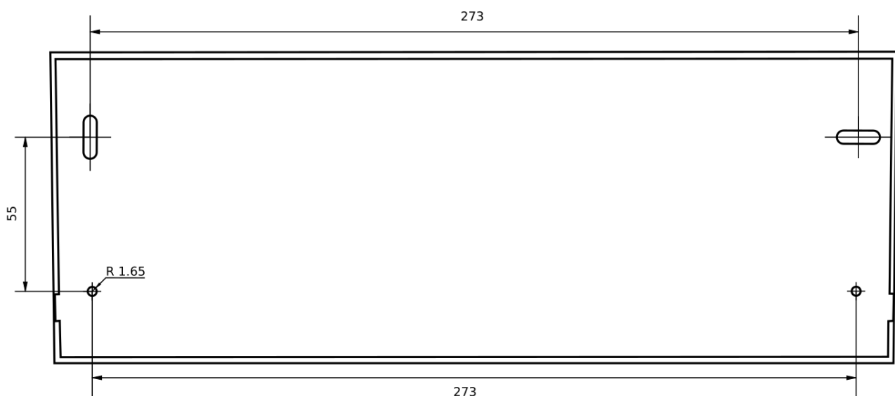
Рисунок 2.4 Монтажные размеры
