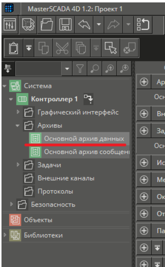
Рисунок 27.2. Фрагменты окна среды разработки MasterSCADA 4D с элементами настройки архива (дерево объектов слева и настройки архивирования справа). Архивирование производится по изменению на внешнюю SD-карту.
