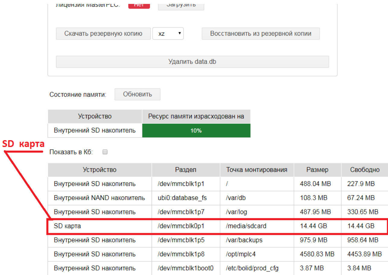
Рисунок 26.3. Сервисное обслуживание вкладка «MPLC» нижняя часть. В контроллер установлена внешняя SD-карта памяти.
