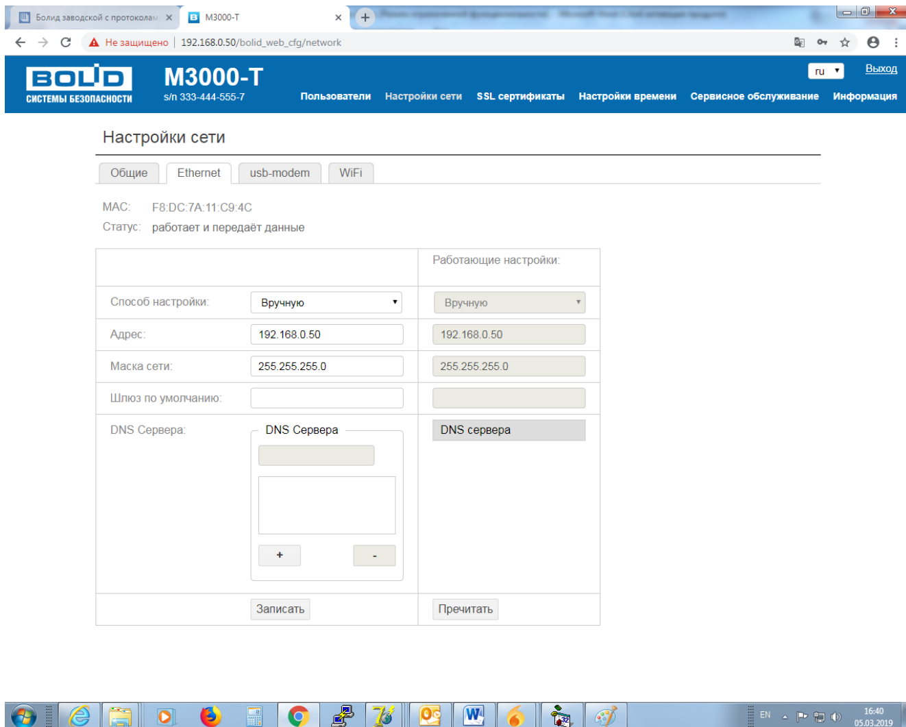
Рисунок 4. Настройка сети, вкладка «Ethernet»
