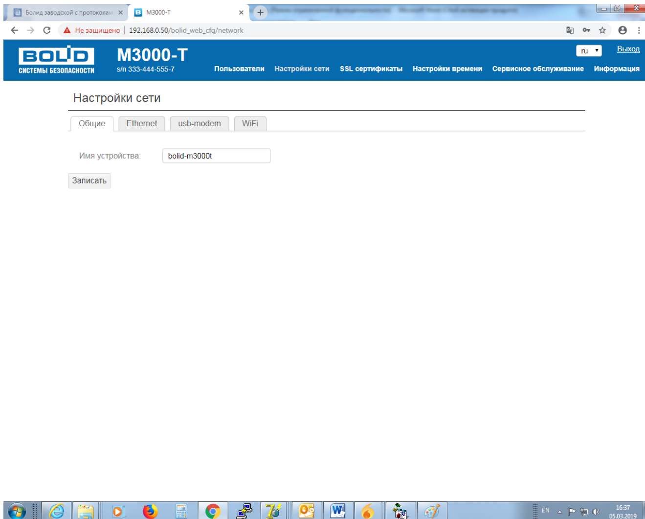
Рисунок 3. Настройка сети
