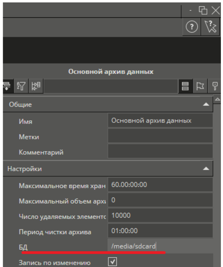
Рисунок 27.2. Фрагменты окна среды разработки MasterSCADA 4D с элементами настройки архива (дерево объектов слева и настройки архивирования справа). Архивирование производится по изменению на внешнюю SD-карту.
