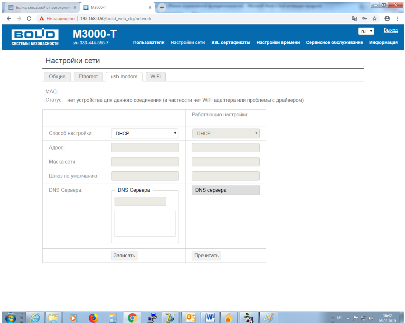
Рисунок 5. Настройка сети, вкладка «usb-modem»
