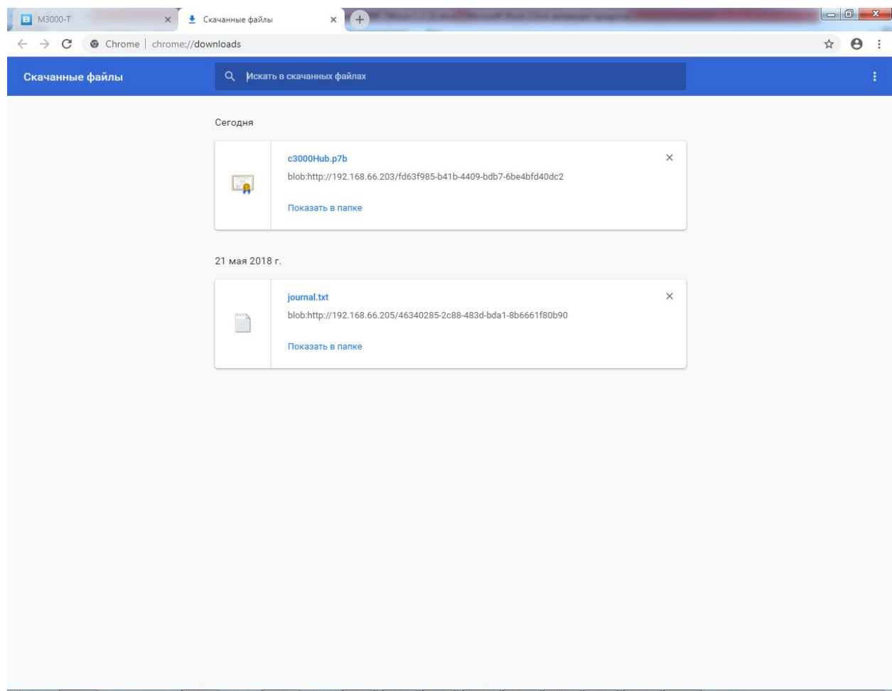
Рисунок 10. Папка загрузок
