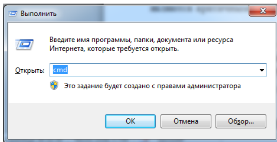
Рисунок 35. Окно «Выполнить»
