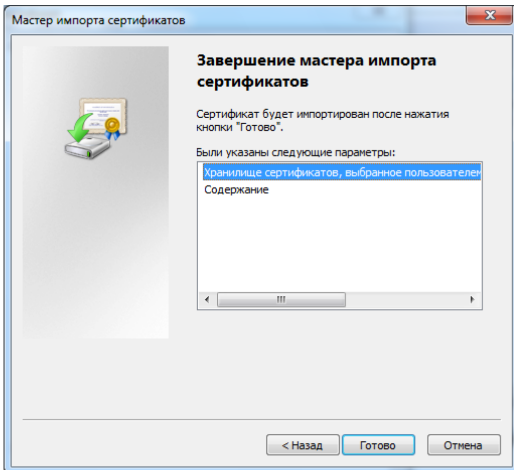
Рисунок 15. Завершение импорта
