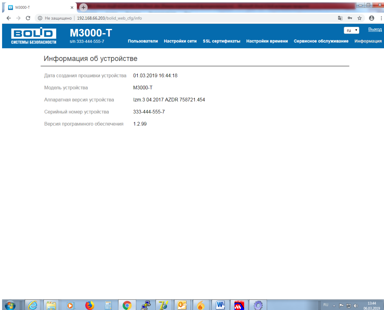
Рисунок 33. Страница «Информация»
