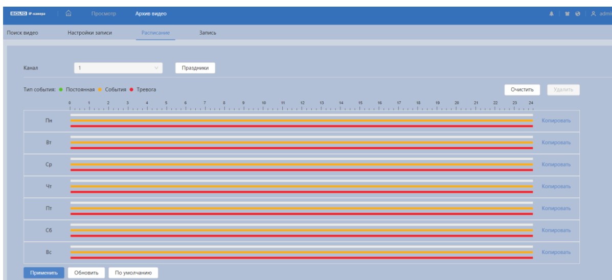
Рисунок 7.124 – Вкладка «Расписание»
