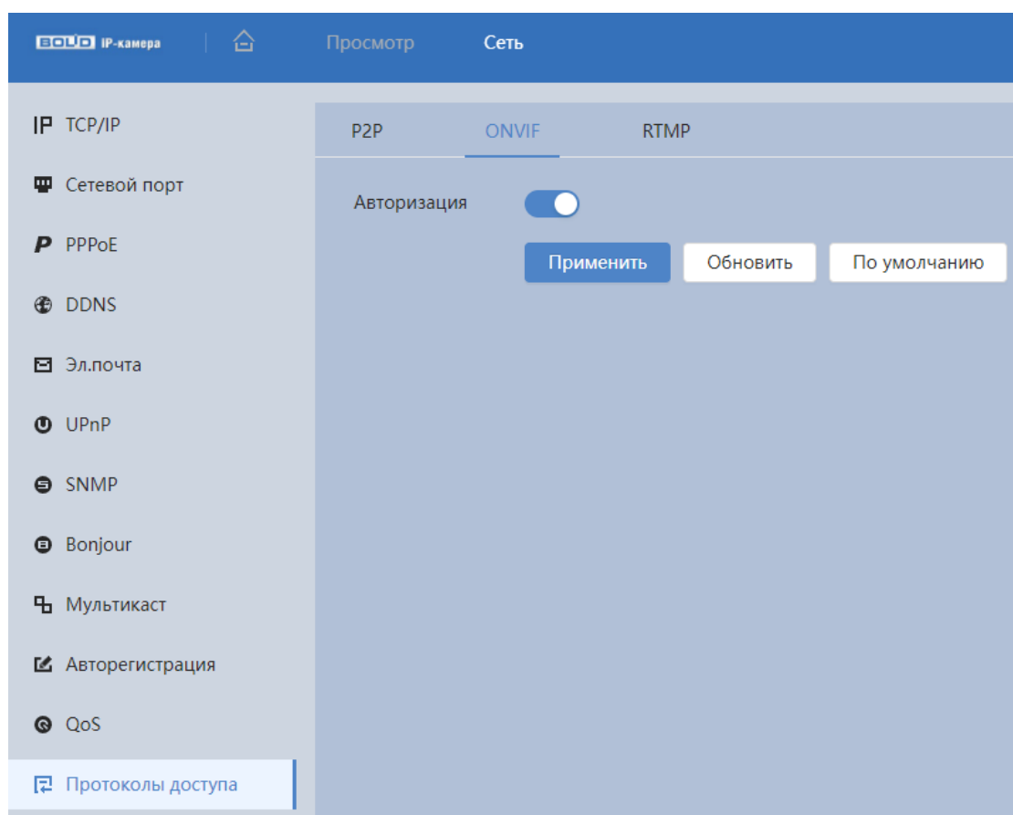
Рисунок 8.20 – Вкладка «ONVIF»
