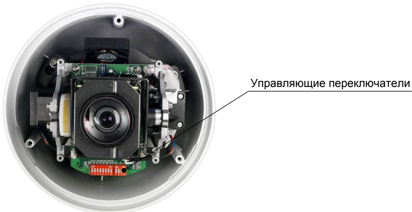
Рисунок 4.2 – Управляющие переключатели
