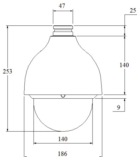
Рисунок 5.1 – Габаритные размеры видеокамеры
